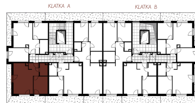
PLAN BUDYNKU
